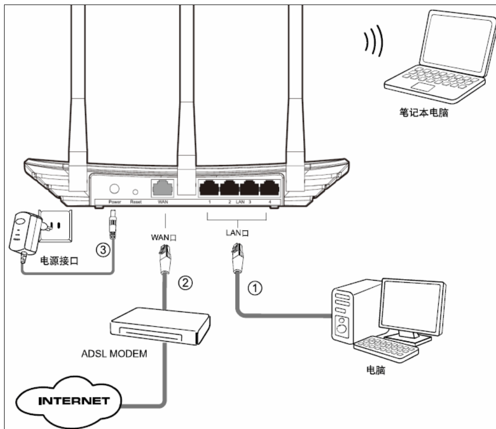
图 4-1 TL-WR880N 硬件安装示意图
